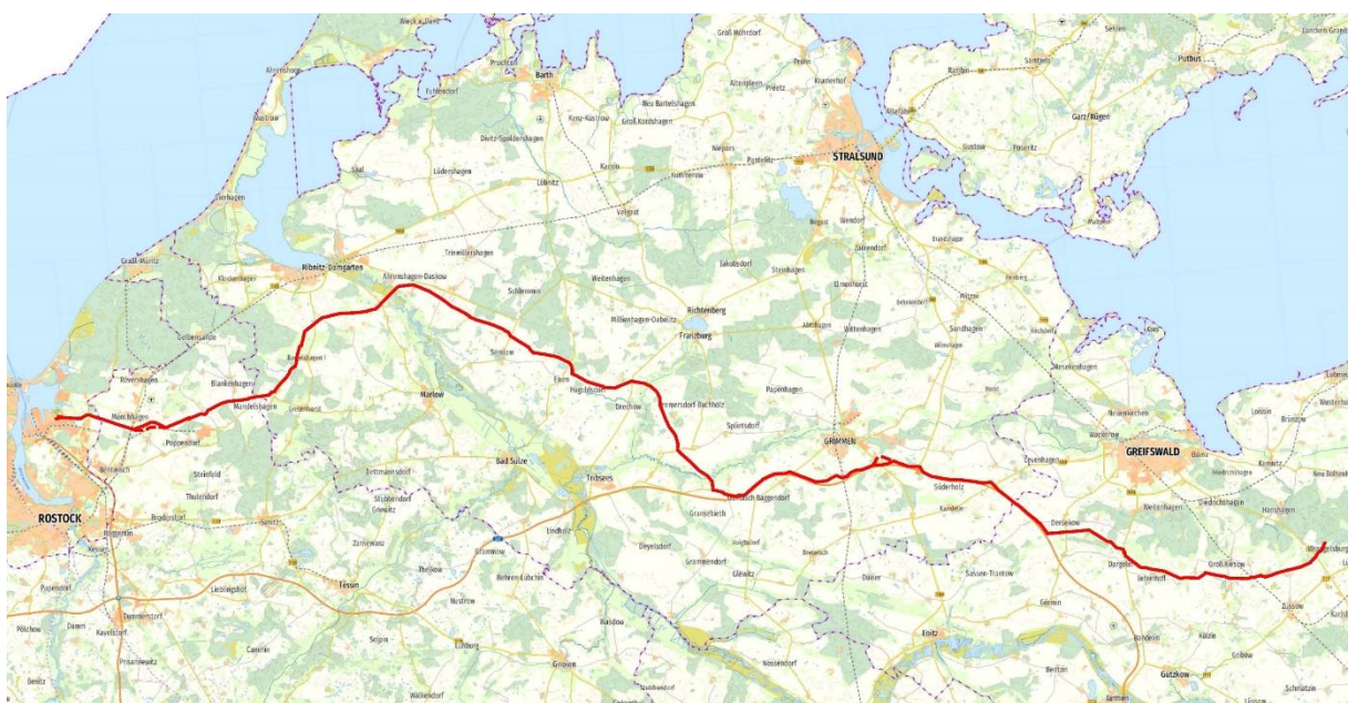
Foto: onmaps.de©GeoBasis-DE/BKG/ZSHH 2024 – Verlauf der HYROW-Wasserstoff-Pipeline
